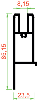
TGT-107 AÇILIR CAM BAZA (TEK CAM) 0.886 KG/M
