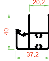
TGI-106 KENET (ISICAM) 0.913 KG/M
