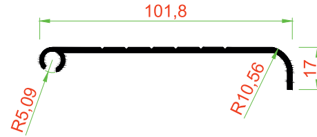
TG-102 KÜPESTE 0.580 KG/M
