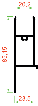
TGI-107 AÇILIR CAM BAZA (ISI CAM) 0.886 KG/M
